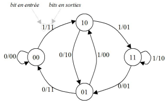
diagramme d'états-transitions
