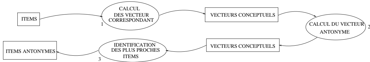
FIG. 1 – parcours des fonctions AntiLex
