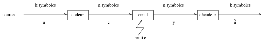
Figure: Transmission avec codage correcteur d'erreur
