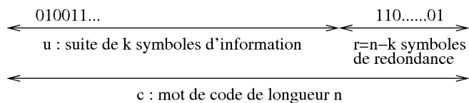
Figure: Formation d'un mot de code par ajout de redondance (code en blocs)
