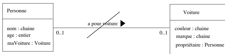
FIG. 1.6 – Schéma de conception pour « a pour voiture »
