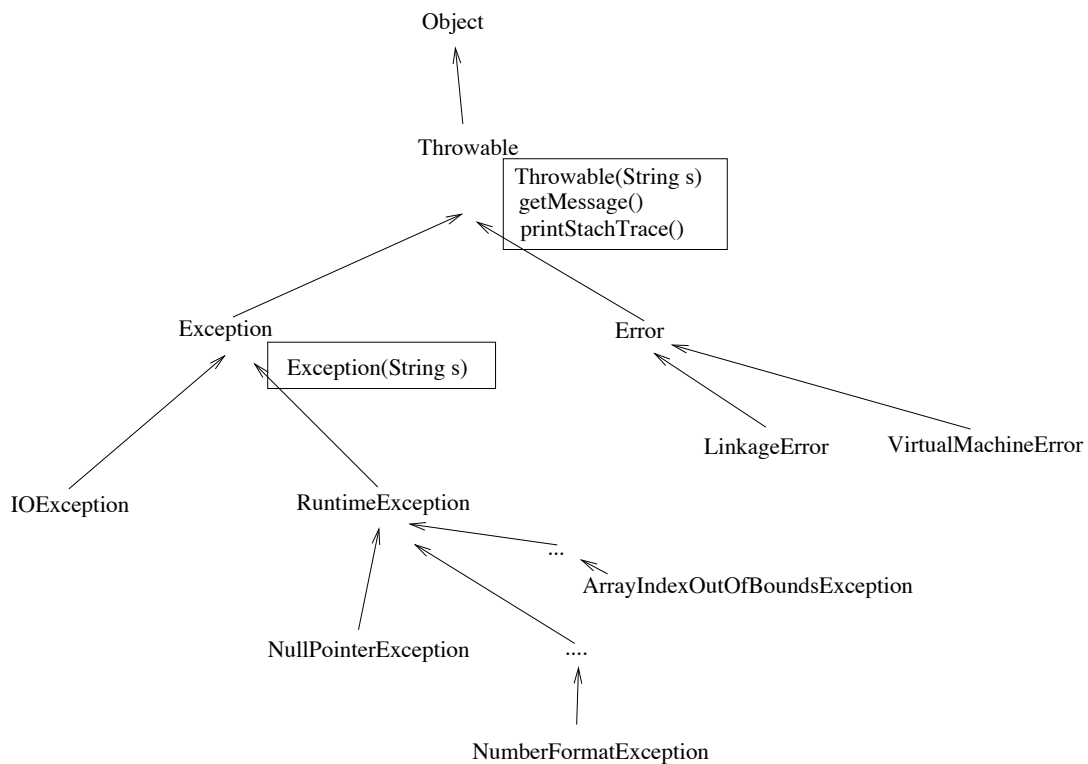
FIG. 6.1 – Les exceptions de Java.
