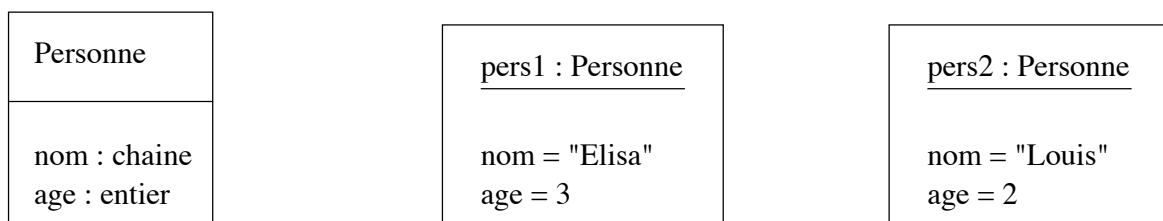
FIG. 1.1 – Une classe Personne et deux instances.
