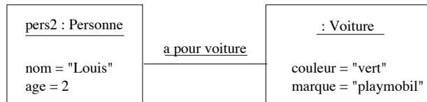
FIG. 1.5 – Personnes et voitures - diagramme d'instances
