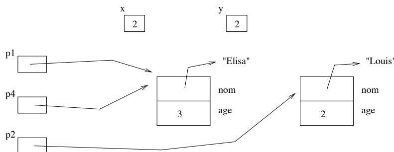
FIG. 1.3 – Désignations et flèches
