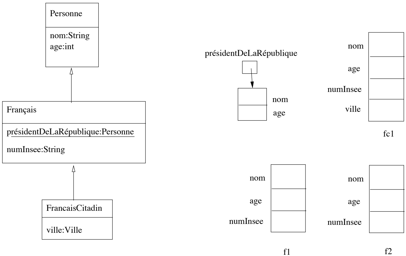
FIG. 5.1 – Variation sur la classe Français.
