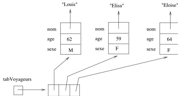
FIG. 3.2 – Un tableau de voyageurs.
