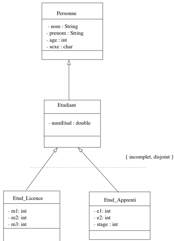
FIG. 4.3 – Une hiérarchie de classes.
