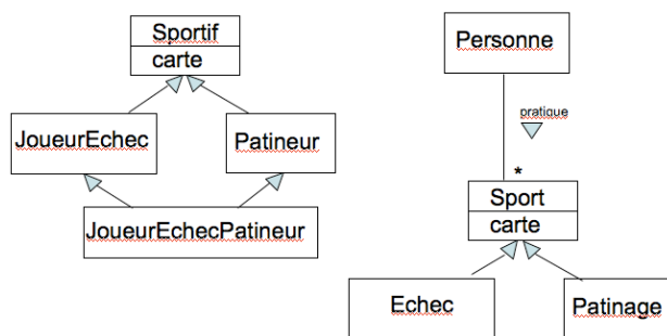
FIG. 8.7 – héritage multiple répété (gauche), solution sans héritage répété (droite)
