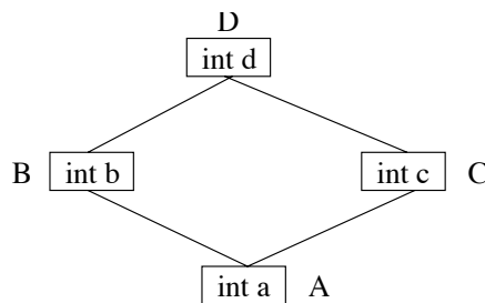
FIG. 8.12 – Situation d’héritage : une instance de A possède-t-elle 1 ou 2 attributs d ?
