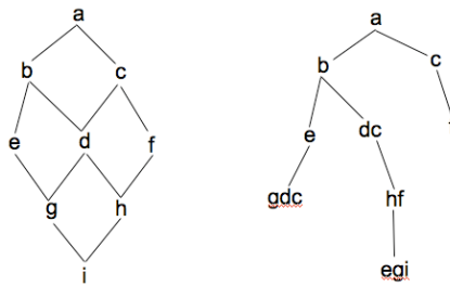
FIG. 8.8 – Structure avec héritage multiple (gauche), héritage simple (droite)
