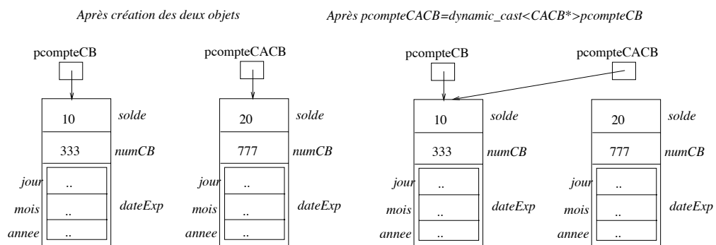
FIG. 3.5 – Affectation entre pointeurs vers des objets
