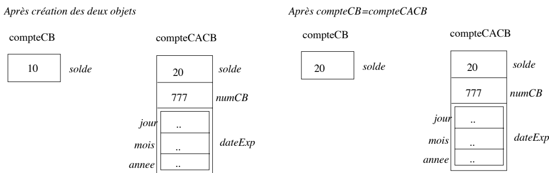
FIG. 3.3 – Affectation entre objets (1)
