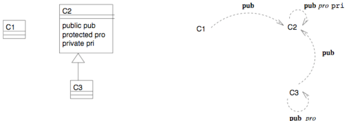
FIG. 10.1 – Accès aux propriétés en dehors d'autres mécanismes. Une flèche de A vers B étiquetée m se lit "dans une méthode de A, on peut envoyer le message m à un objet de type statique B"
