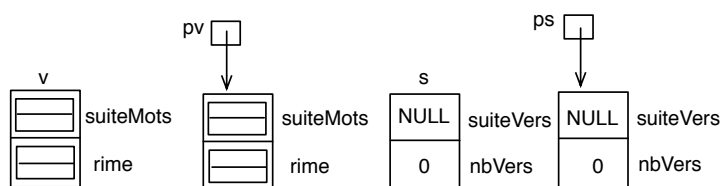
FIG. 2.8 – Structure en mémoire après création des vers et strophes
