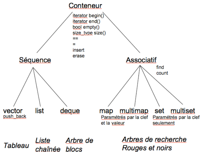
FIG. 7.1 – Les conteneurs avec quelques méthodes
