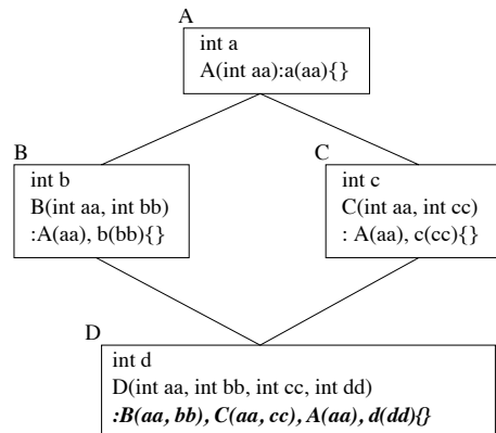
FIG. 8.15 – Passage de paramètres aux constructeurs (héritage virtuel)
