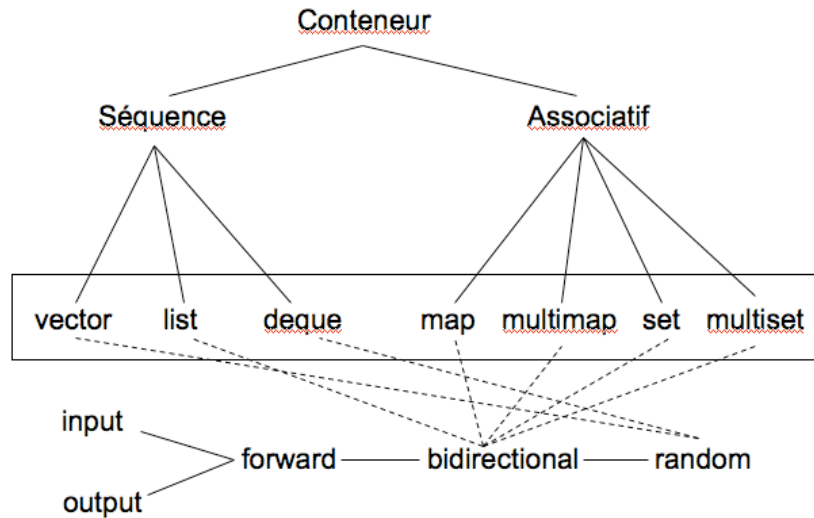
FIG. 7.3 – Les liens entre conteneurs et itérateurs
