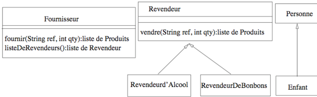
FIG. 10.4 – Un diagramme de classes
