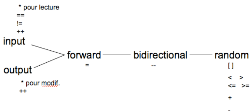
FIG. 7.2 – Les itérateurs et leurs opérations
