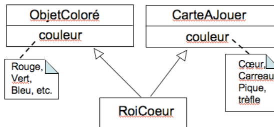
FIG. 8.6 – Situation de conflit de nom
