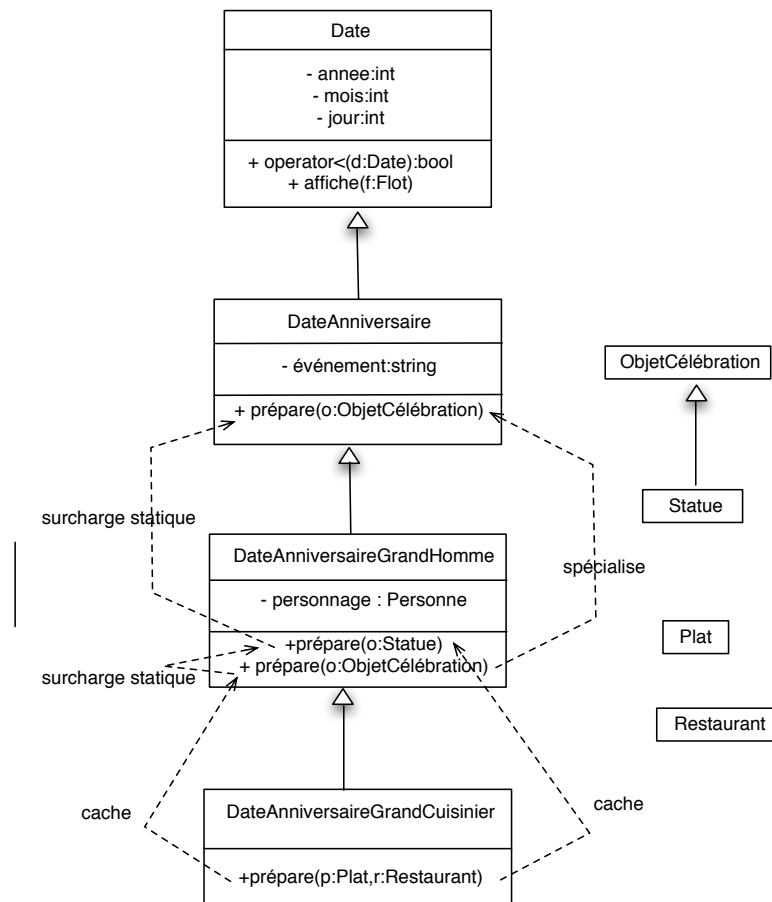
FIG. 4.1 – Schéma de surcharge, définition et masquage
