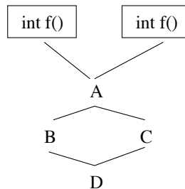
FIG. 8.10 – Désambiguïsation et connaissance de la hiérarchie
