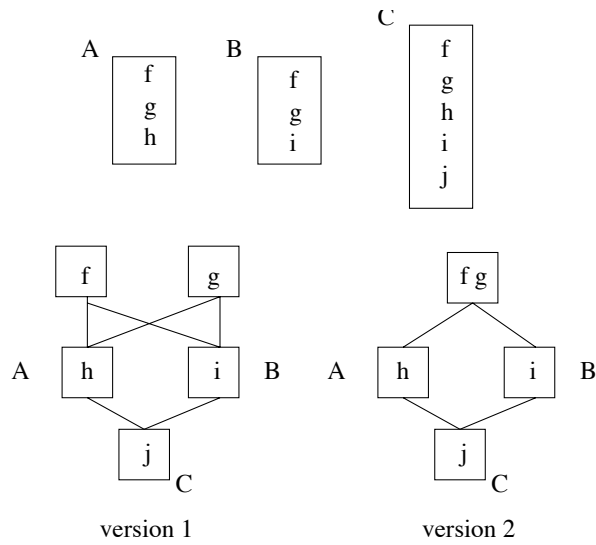
FIG. 8.4 – Trois classes et deux factorisations maximales
