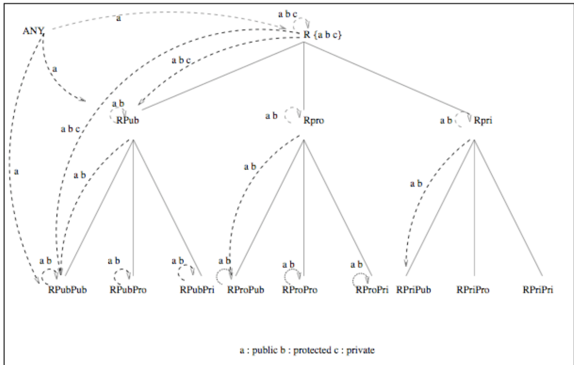
FIG. 10.3 – Accès aux propriétés et protections sur liens d'héritage; C_x est dérivée de C avec la protection x
