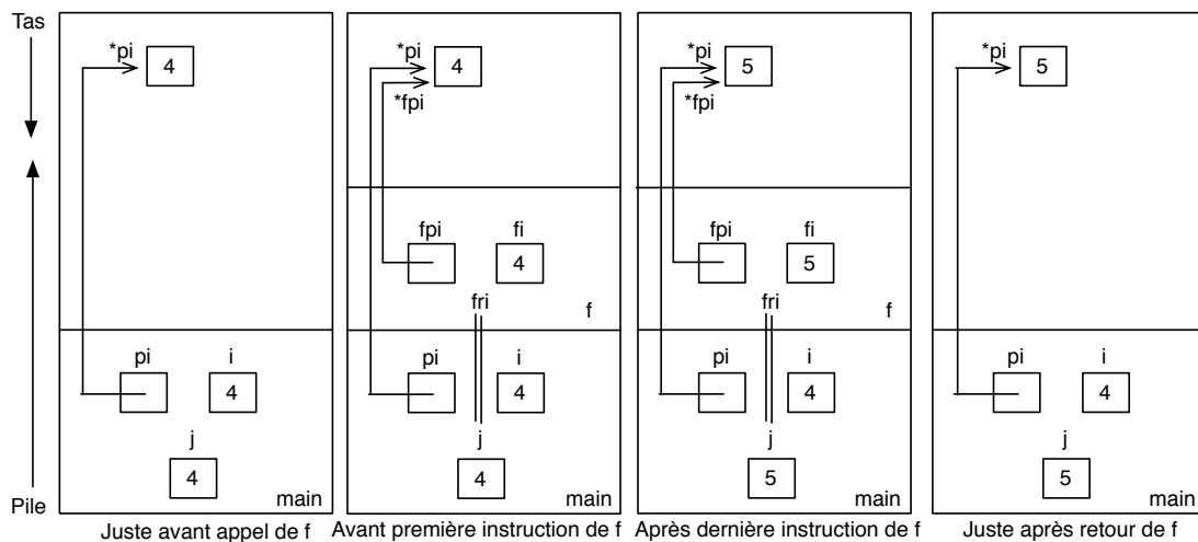
FIG. 2.9 – Evolution de la mémoire lors des passages de paramètres et retour de f
