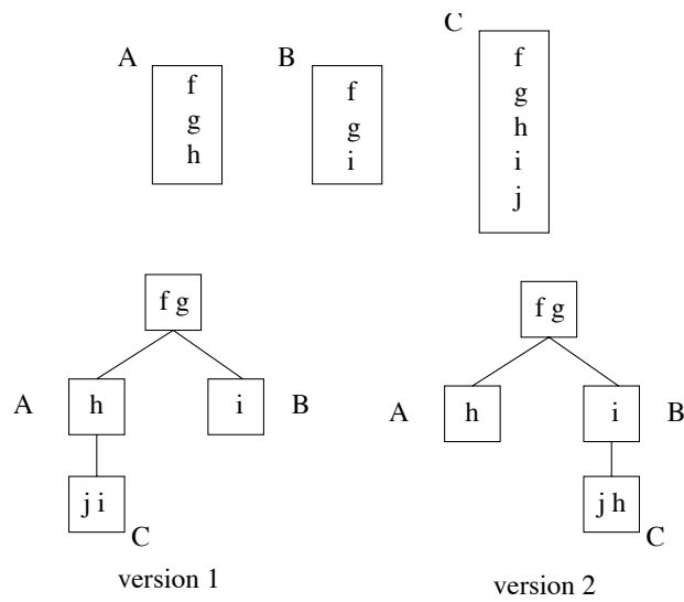
FIG. 8.5 – Trois classes et deux factorisations en héritage simple
