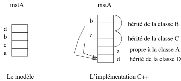
FIG. 8.14 – Situation d’héritage virtuel en C++, vue logique de l’instance
