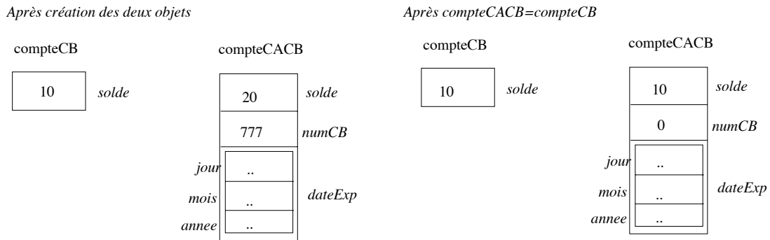
FIG. 3.4 – Affectation entre objets (2)
