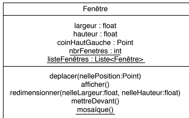
FIG. 5.1 – La classe Fenetre en UML
