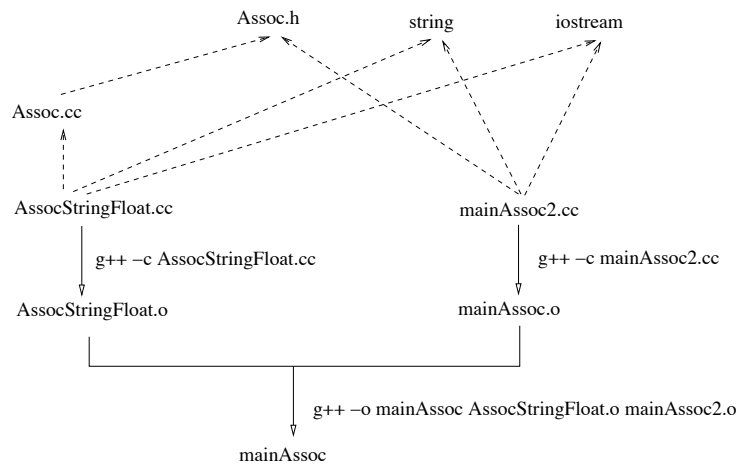
FIG. 6.2 – Un exemple de compilation et d'édition de liens avec instantiation séparée
