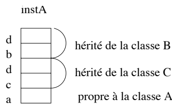
Désignation des attributs, B::d, C::d
