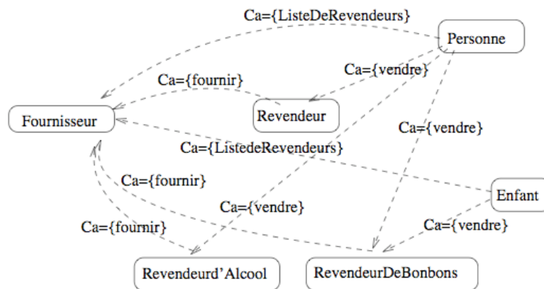
FIG. 10.4 – Un diagramme de classes
