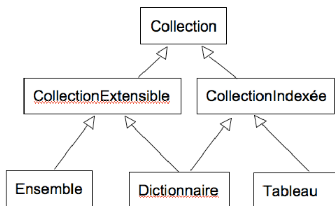
FIG. 8.2 – multi-classification de quelques collections
