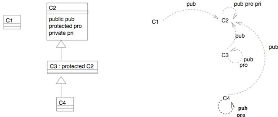
FIG. 10.2 – Accès aux propriétés avec protected sur un lien d'héritage
