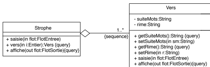
FIG. 2.1 – Éléments de la représentation des strophes
