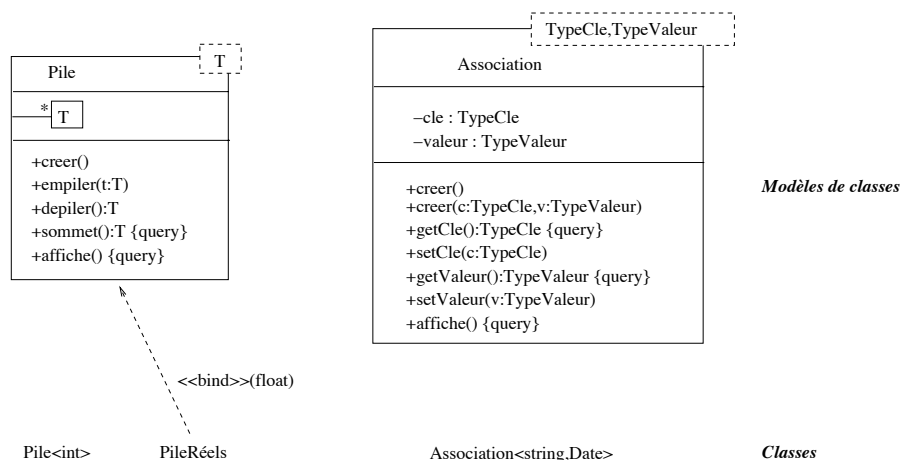
FIG. 6.1 – Modèles de classes et leurs instantiations notés en UML
