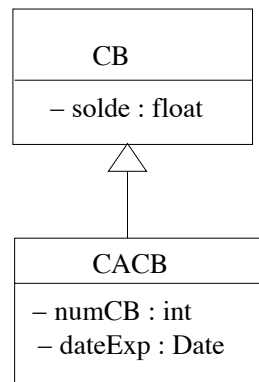
FIG. 3.1 – Comptes bancaires simplifiés
