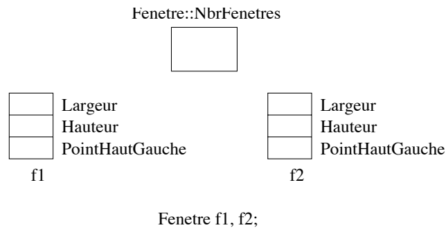
FIG. 5.2 – Fenêtres graphiques
