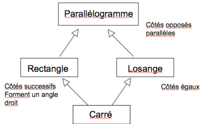
FIG. 8.1 – multi-classification de quelques polygones
