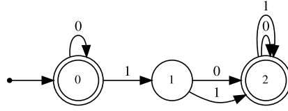
Fig. 2. Walnut output automaton
