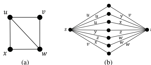
Figura 4: (a) O grafo G e (b) seu (s, t) -grafo G' .
