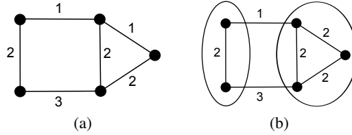
Figura 1: (a) Um grafo aresta-colorido G e (b) Um corte de G com capacidade 2.
