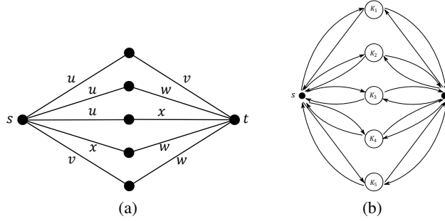
Figura 7: (a) Grafo G' usado na redução de VERTEX COVER e (b) o digrafo G'' .
