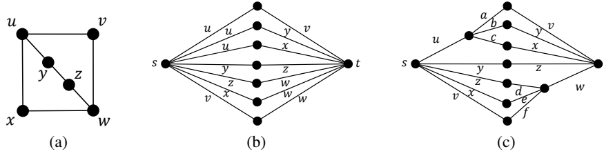
Figura 6: (a) O grafo G , (b) seu (s, t) -grafo G' e (c) G''
