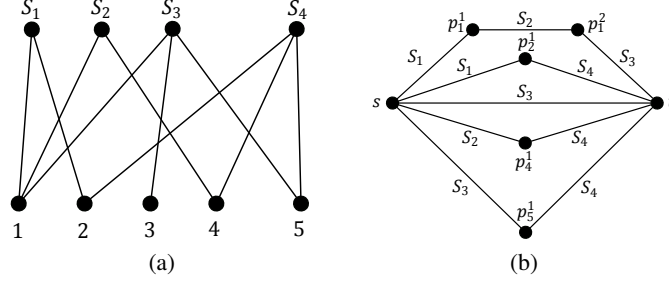
Figura 3: (a) Grafo bipartido G' usado na redução de SET COVER e (b) o (s, t) -grafo G^c .
