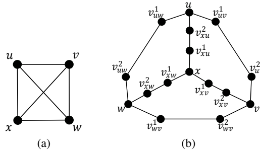
Figura 5: (a) Um grafo cúbico G e (b) seu grafo associado G' .
