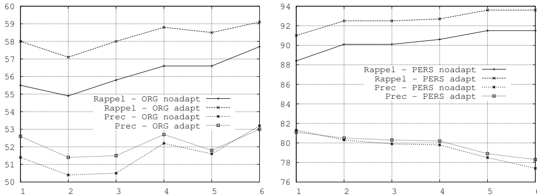
FIG. 1 – Courbes d'apprentissage de LIANE sur les catégories PERS et ORG en fonction du volume des données d'apprentissage issues du corpus étiqueté par NP. Les résultats sont donnés avec et sans adaptation lexicale.
