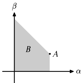
Рис. 14.3. Параметры гипотезы A и её «упрощения» B
