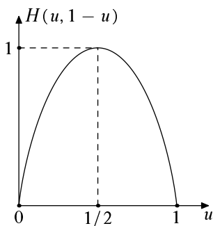
Рис. 3.1. Шенноновская энтропия как функция u .
