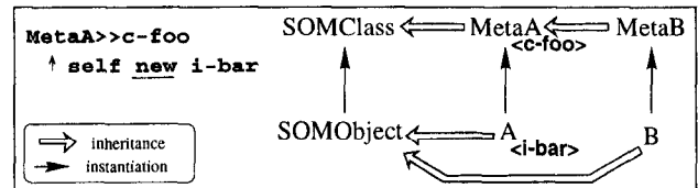
Figure 6: SOM downward compatibility failure example
