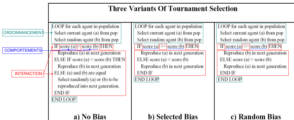
FIG. 7.1 – Identification du code lié à l'interaction dans [Edmonds &amp; Hales, 2003].
