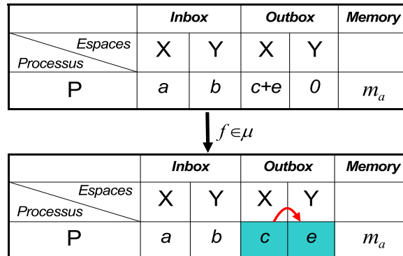
FIG. 8.4 – Application d'une loi de mouvement entre deux espaces d'interaction.
