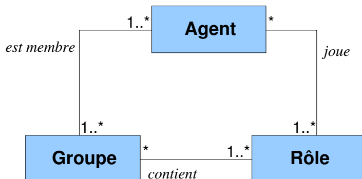
FIG. 5.1 – Le modèle Agent Groupe Rôle.
