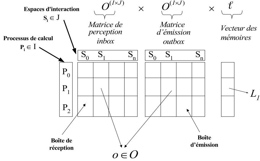
FIG. 8.2 – La structure statique d'un environnement MIC* : un triplet de matrices.
