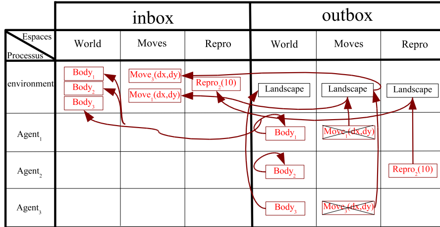
FIG. 9.4 – Evolution du terme MIC* après l'application de envPerception_{\mathcal{T}} .
