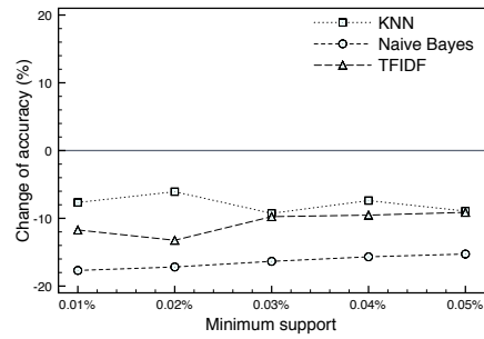
(d) Top-10 frequent words pruned.
