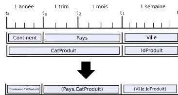
Figure 8 – Résultat de l'intersection des fonctions de précision
