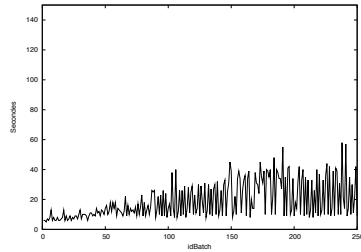
(b): Temps vs degré 5 (D5L3B250T20)
