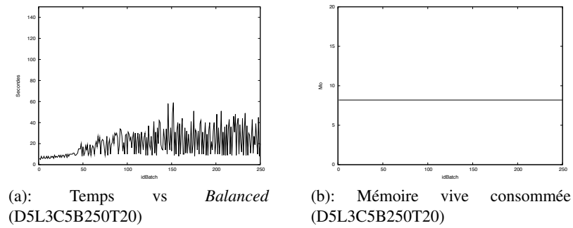
Figure 11 – Influence des fonctions de précision (2/2)
