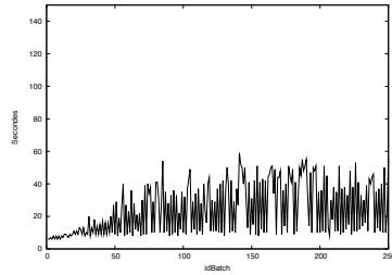
(a): Temps vs 10 dimensions (L3C5B250T20)
