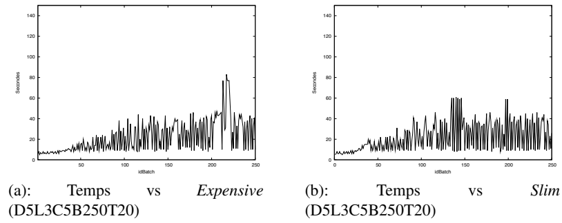
Figure 10 – Influence des fonctions de précision (1/2)
