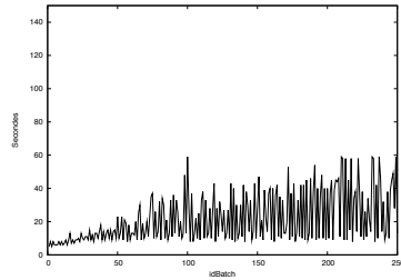
(a): Temps vs profondeur 5 (D5C5B250T20)
