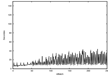
(a): Temps vs profondeur 3 (D5C5B250T20)
