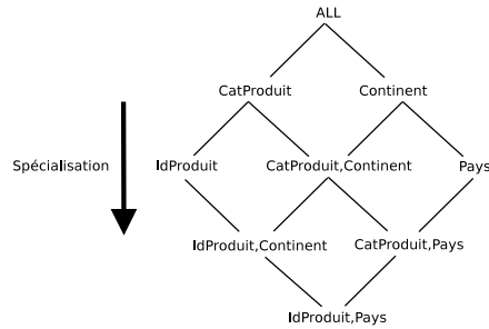
Figure 2 – Exemple de treillis
