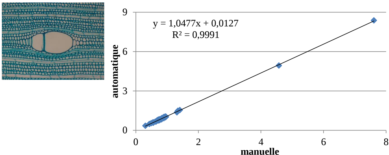
Figure 26. Etude de la surface de bassin chez l'acajou ( Pycnanthus sp. ). En abscisse, les surfaces normalisées obtenues à partir d'une segmentation manuelle. En ordonnée, celles obtenues à partir de la méthode automatique. Le coefficient de détermination est proche de 1, montrant un bon ajustement des surfaces.
