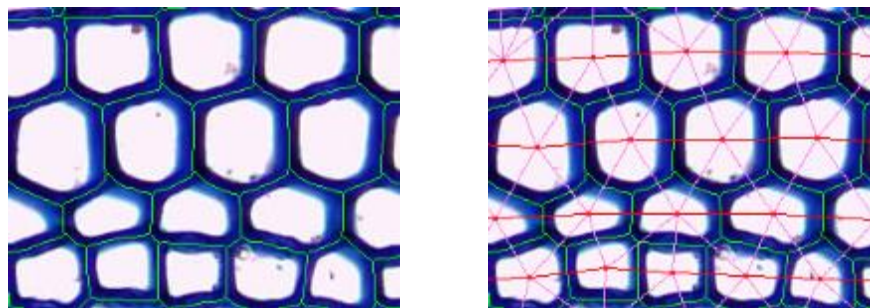
Figure 20. A gauche : les lignes de crête, représentées en vert, produites par le watershed correspondant globalement à la lamelle moyenne, l'espace entre les parois cellulaires ; les bassins sont une bonne approximation des cellules. A droite : le graphe d'adjacence des cellules est construit à partir des lignes de crête ; les chemins correspondant aux files cellulaires sont affichés en rouge.
